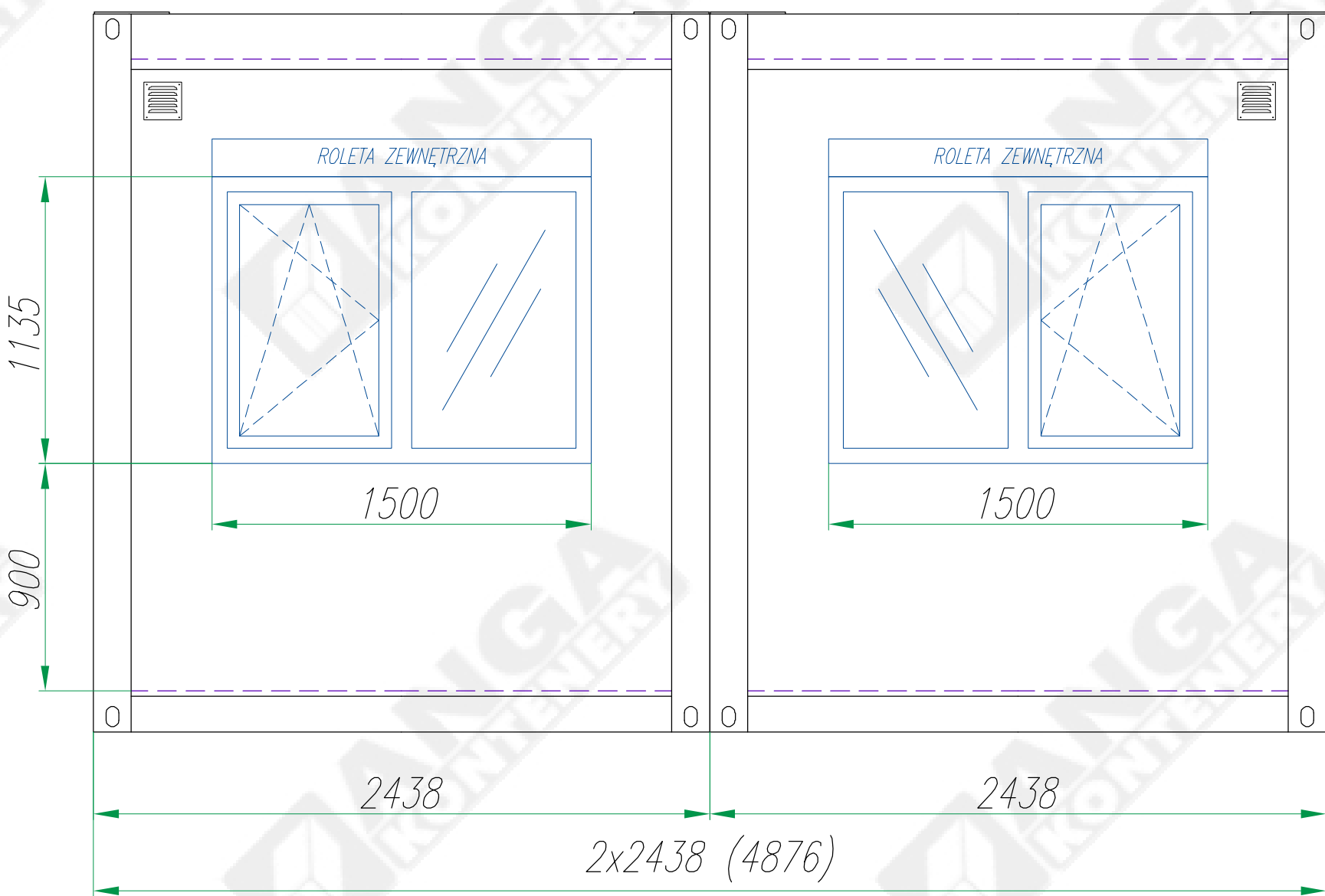
Widok C
