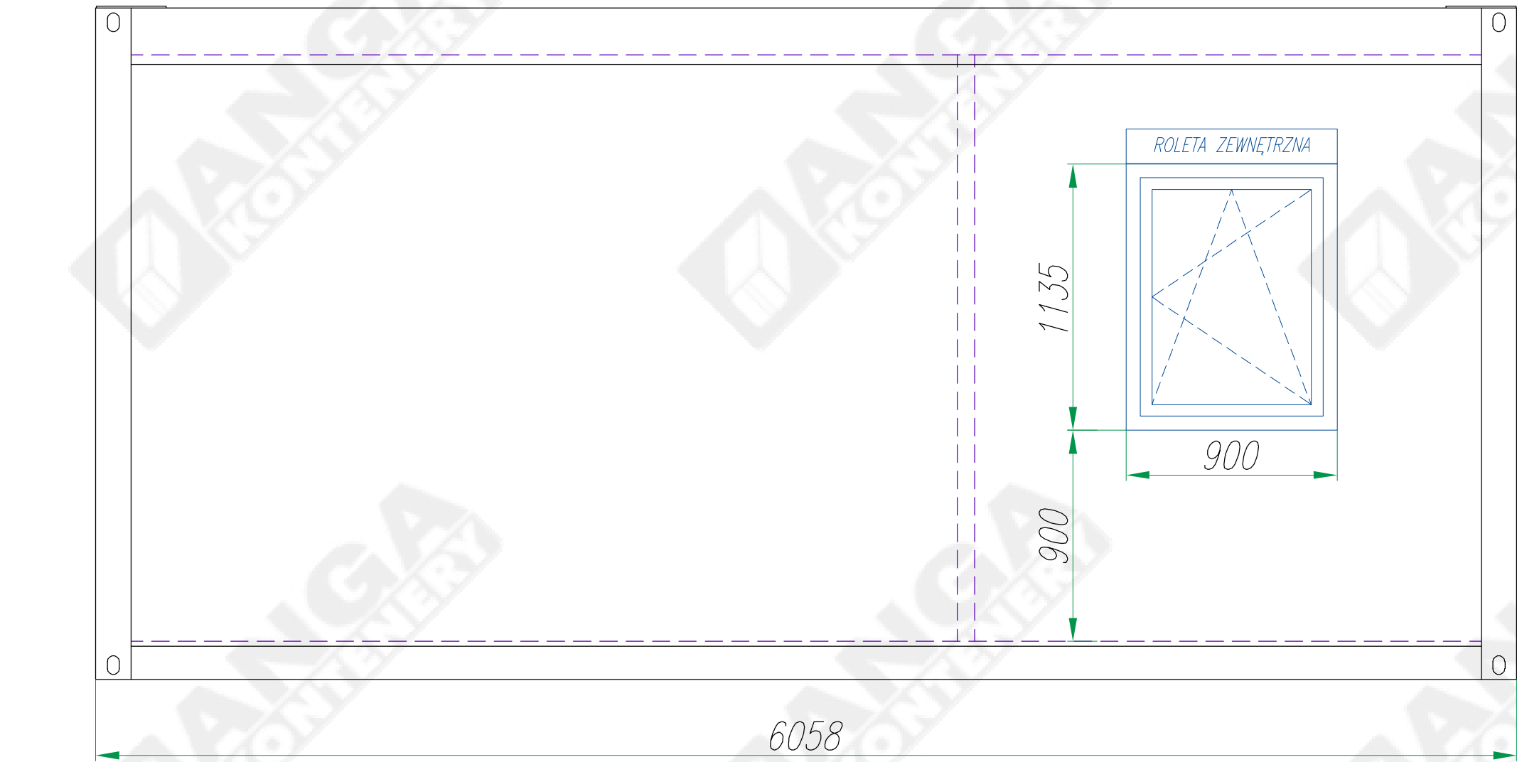
Widok A
